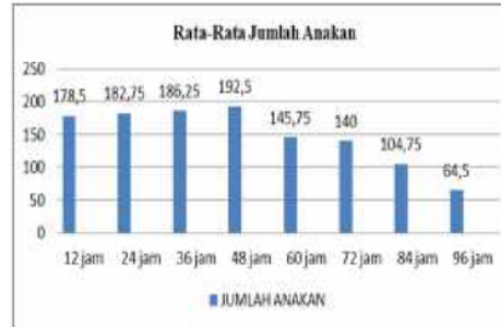
Gambar 1. Histogram rata-rata umlah anakan pada berbagai umur betina D. melanogaster Strain Tx
